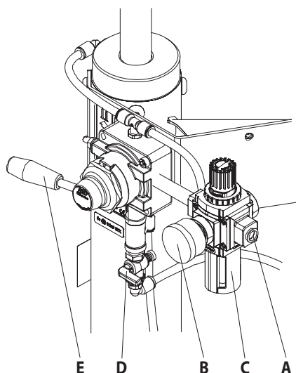
Modèle RM552H-BXX-XX
